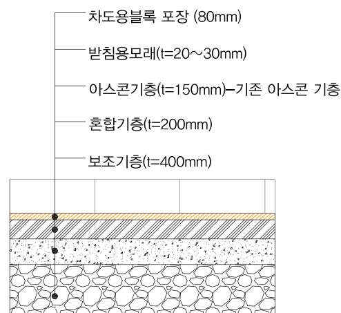
아스콘 포장
