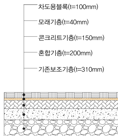
콘크리트기층 포장
